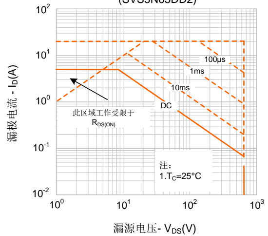
图 9-2. 最大安全工作区域 (SVS5N65DD2)
