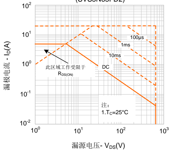
图 9-1. 最大安全工作区域 (SVS5N65FD2)
